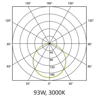
93W, 3000K
